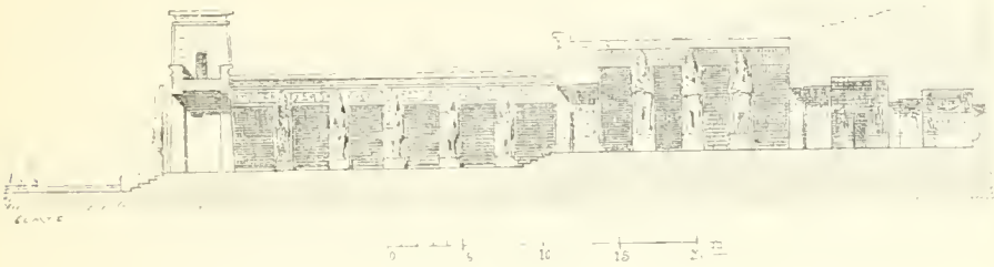
FIG. 239.—Gherf-Hosseini, longitudinal section ; from Prisse.
