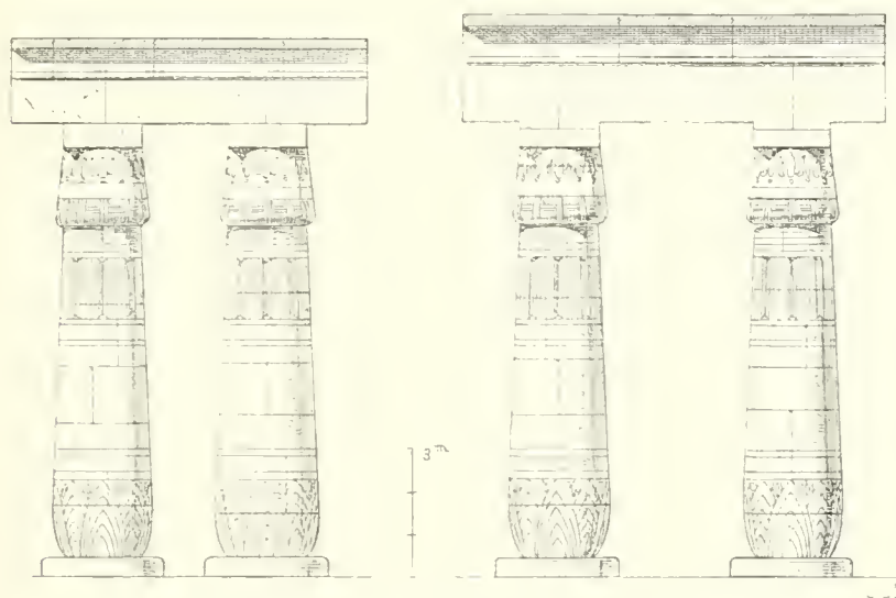
FIG. 66.—Ramesseum, Thebes. ( Description de l'Égypte , t. ii., pl. 28.)
