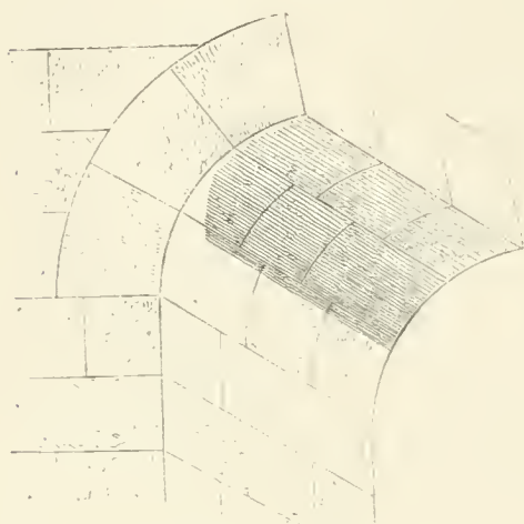
FIG. 78.—Arrangement of voussoirs.
