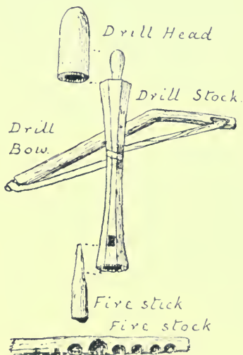
91. FIRE APPARATUS. 1:10.
